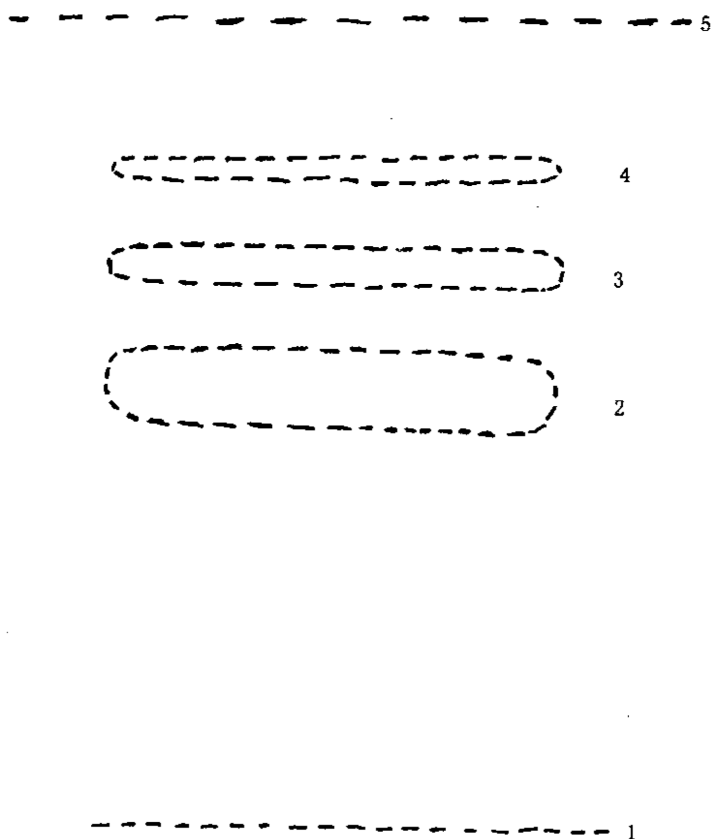
1—原点;2—异丙威谱带 R_f=0.59 ;3—邻异丙基酚;4—其他杂质;5—溶剂前沿
